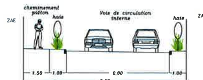
Profil en travers type :
